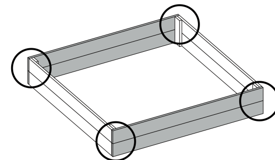
Przykręć deski przy pomocy 16 wkrętów W1, po 4 wkręty na każdym z 4 rogów.
