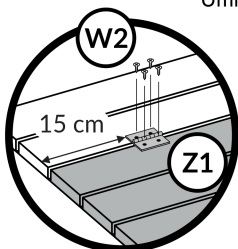
Przykręć 4 zawiasy Z1 w odległości 15 cm od krawędzi, przy pomocy 16 wkrętów W2, po 4 wkręty na każdy z 4 zawiasów.
