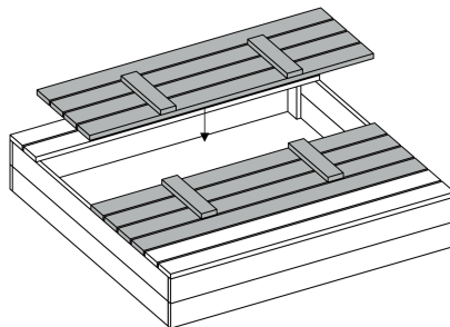
Połącz ławeczki z ramą. Umieść ławeczki na wierzchu ramy, zawiasami do dołu.
