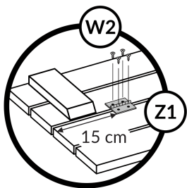
Przykręć 4 zawiasy Z1 w odległości 15 cm od krawędzi, przy pomocy 16 wkrętów W2, po 4 wkręty na każdy z 4 zawiasów.
