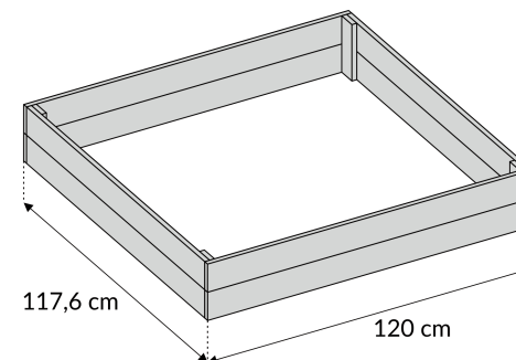
Przykręć deski przy pomocy 16 wkrętów W1, po 4 wkręty na każdym z 4 rogów.
