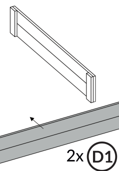
Otrzymane wcześniej 2 boki połącz na szczytach 4 deskami D1, po 2 z każdej strony.
