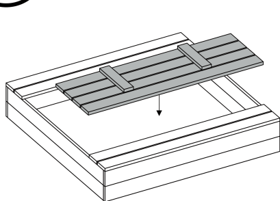
Połącz ławeczki z ramą. Umieść ławeczki na wierzchu ramy, zawiasami do dołu.
